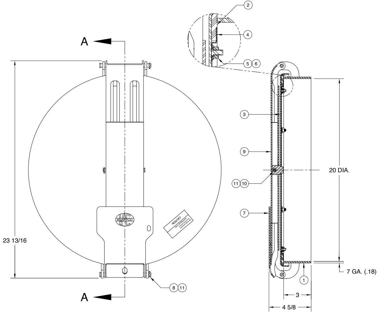
SECTION A-A
