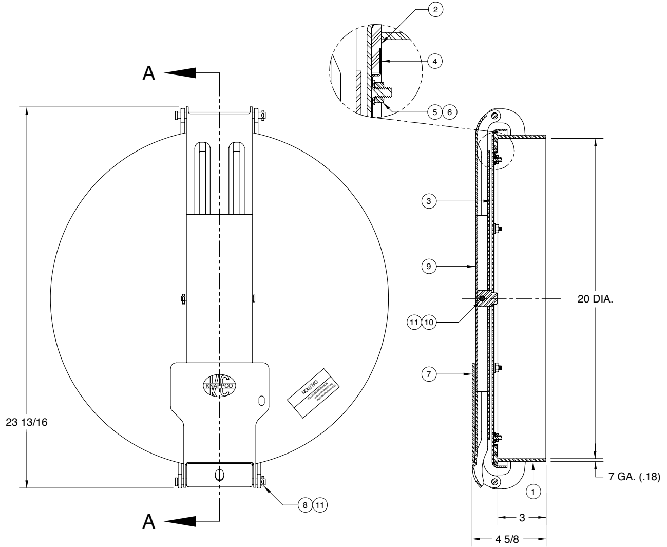
SECTION A-A
