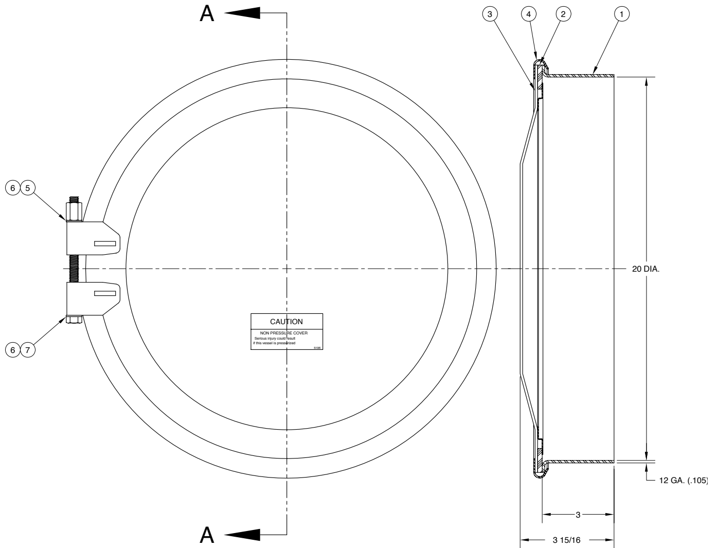
SECTION A-A
